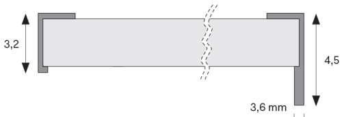
SEZIONE ANTA DOOR SECTION
